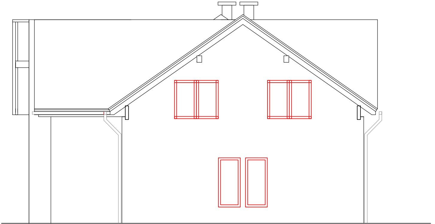
SEVERNA FASADA
