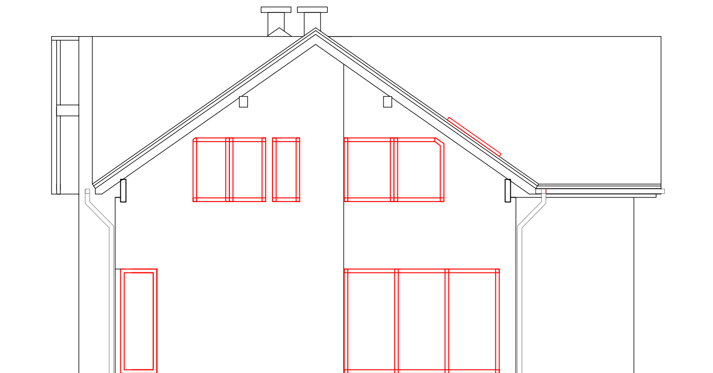
JUŽNA FASADA
