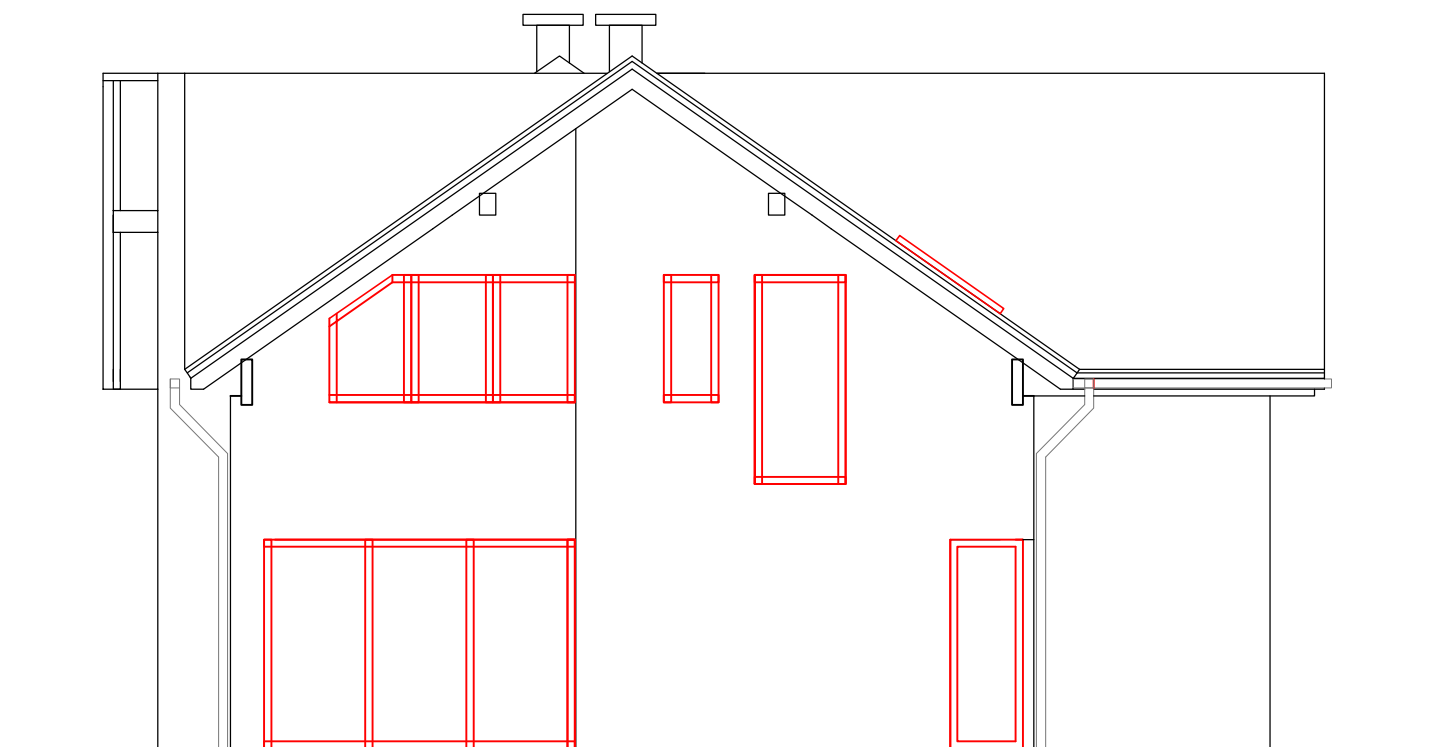
SEVERNA FASADA
